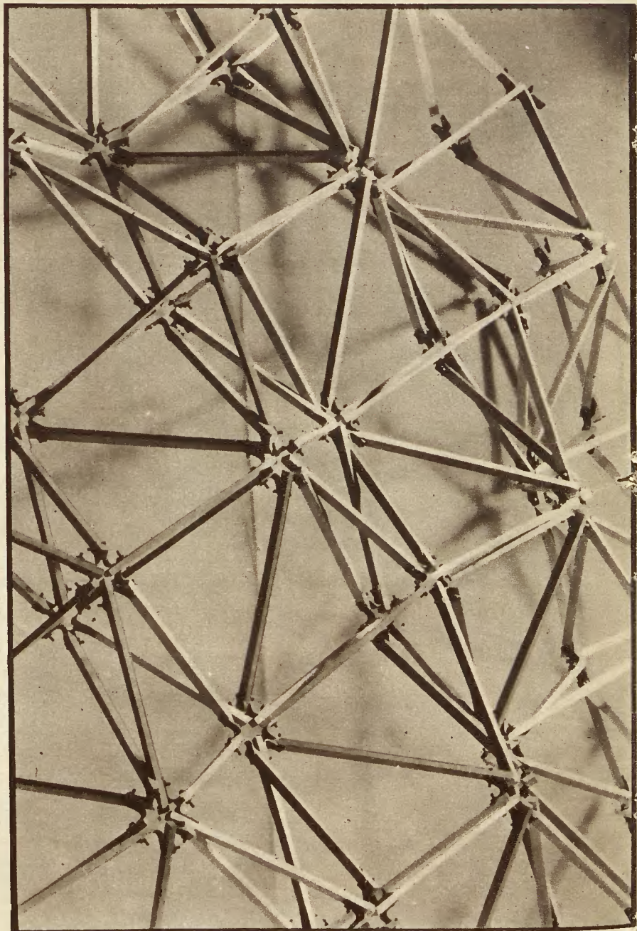
Struktur in drei Dimensionen. Ingenieur: Le Ricólais
