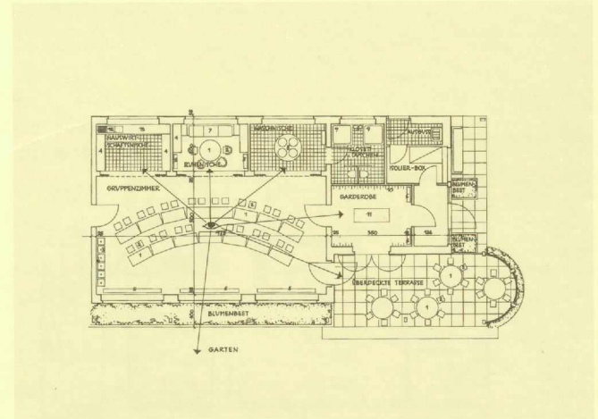
Plan Nr. 5: Raumelement für 1 Kindergruppe – Typ 4
