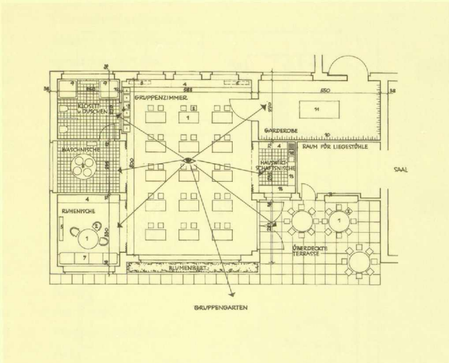
Plan Nr. 1: Raumelement für 1 Kindergruppe – Typ 1
