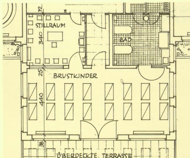
Plan Nr. 9: Raumelement für die Gruppe der Brustkinder in Krippen
