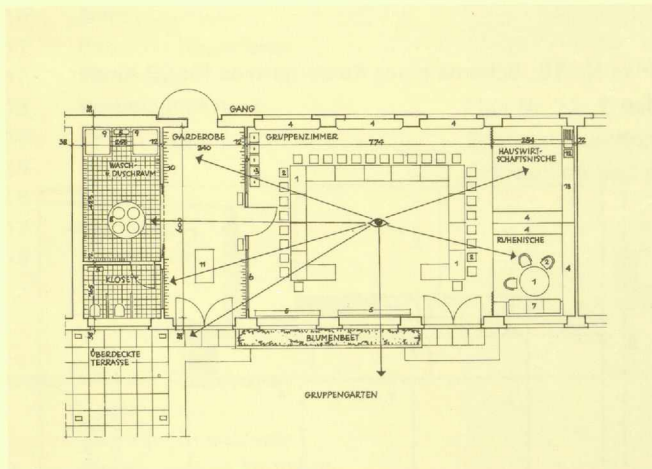
Plan Nr. 4: Raumelement für 1 Kindergruppe – Typ 3
