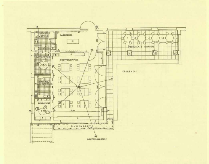
Plan Nr. 3: Raumelement für 1 Kindergruppe – Typ 2
