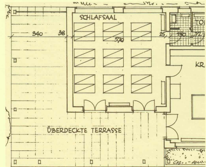
Plan Nr. 10: Raumelement für die Gruppe der Kriech- und Laufkinder
