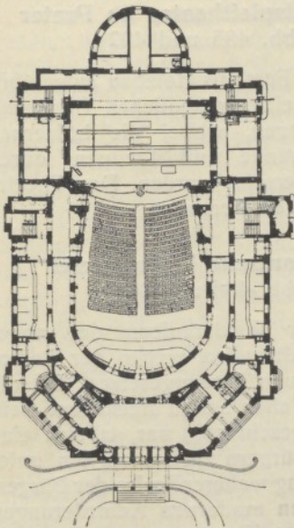
Abb. 486. Deutsches Volkstheater. Parterre. 1:1000.
