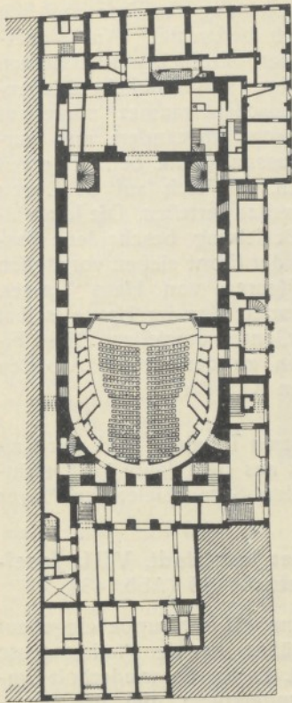
Abb. 482. Theater an der Wien. Parterre. 1:1000.
