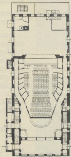
Abb. 485. Lustspieltheater im Prater. Parterre. 1:1000.
