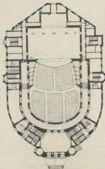
Abb. 488. Jubiläumstheater. Parterre. 1:1000.
