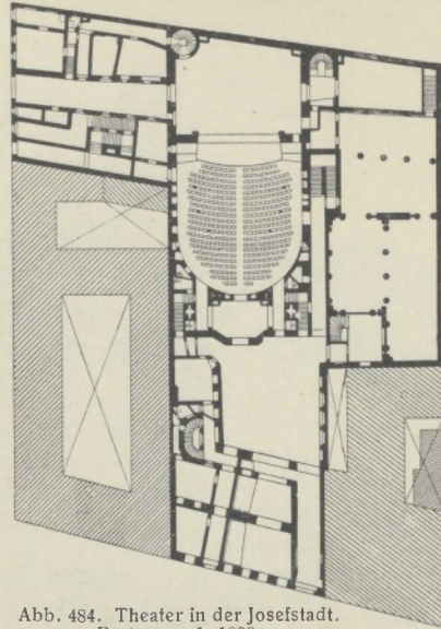
Abb. 484. Theater in der Josefstadt. Parterre. 1:1000.
