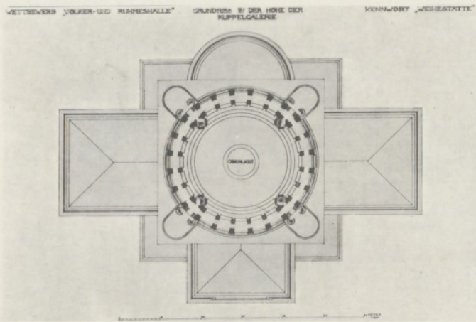
Nr. 1. Kennwort: — Weihestätte. — Karl Troll, Architekt (Atelier Troll und Stoppel).
