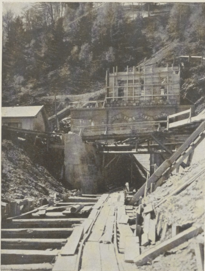
Bau des Wasserschlosses beim Arthurkraftwerk der Mitterberger Kupfer A. G.
