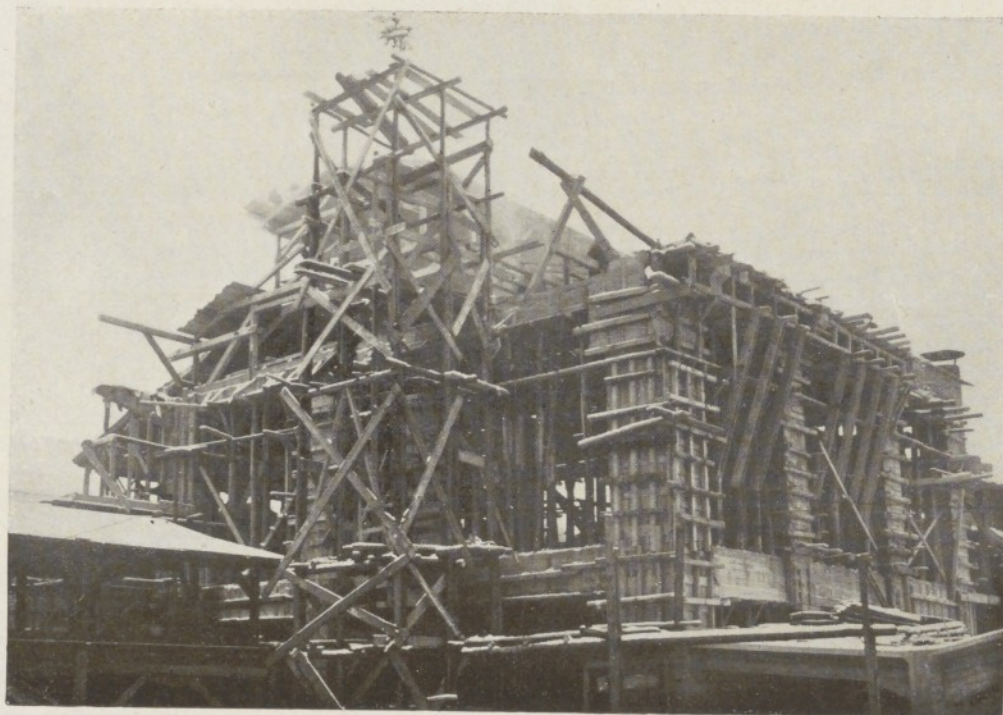
Bau einer Schachtofen-Anlage.
