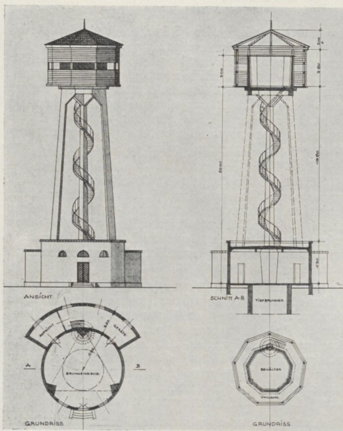
Hochreservoir für die Wasserleitung in Wieselburg.
