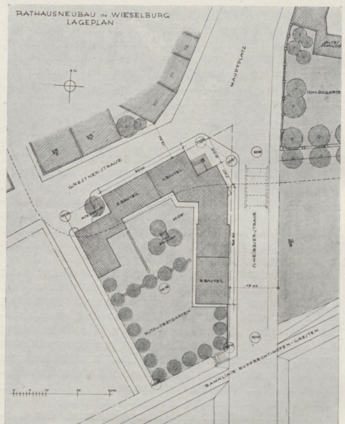
Lageplan des Rathausneubaues in Wieselburg.
