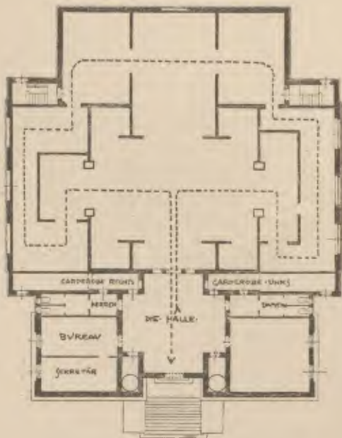
ORIENTIRVNGSPLAN DES AVSSTELLVNGSGEBÄVDES WIENZEILE 2.
