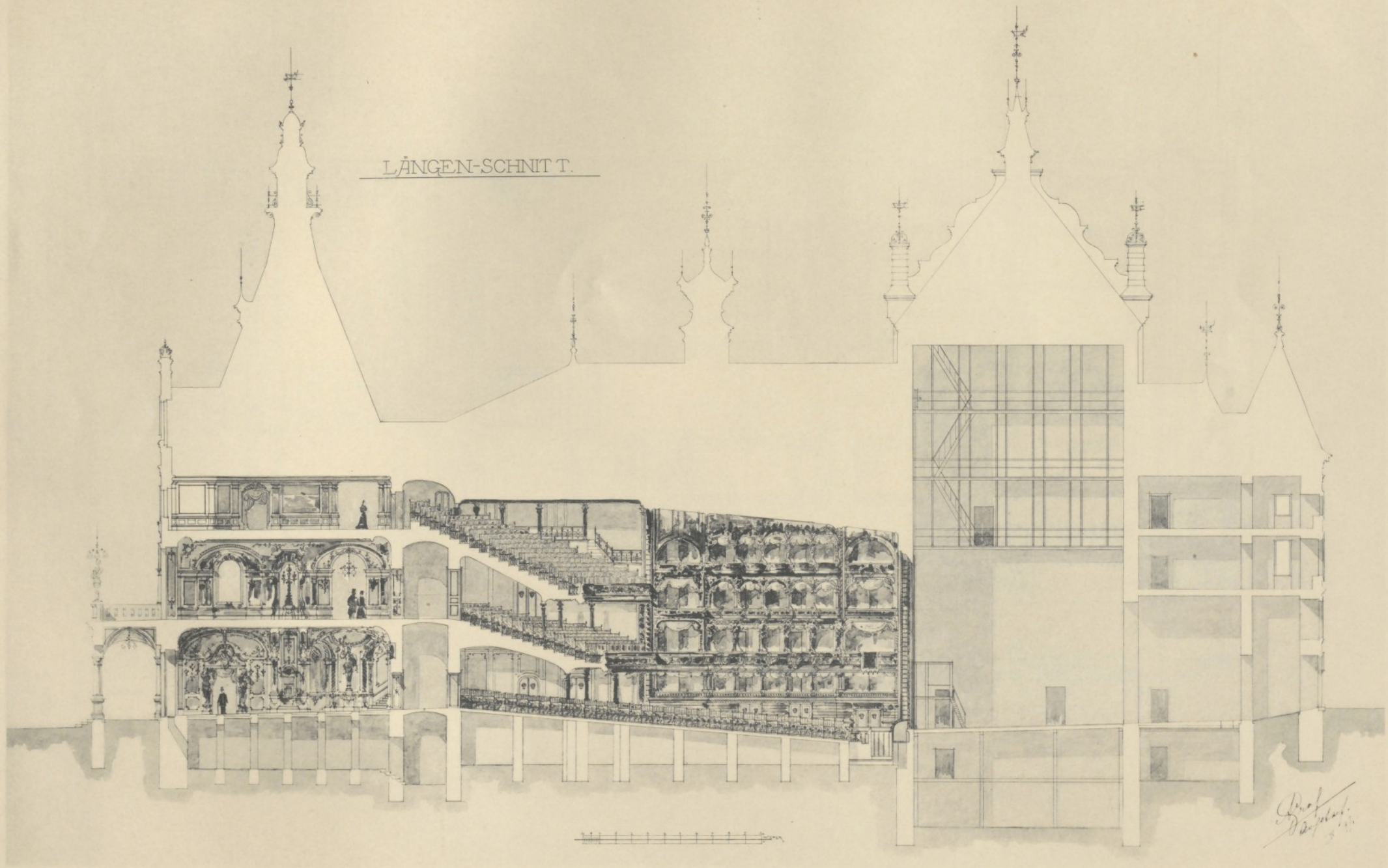
ENTWURF ZUM KAISER-JUBILÄUMS-STADT-THEATER IN WIEN. ARCHITEKT A. GRAF, WIEN.
