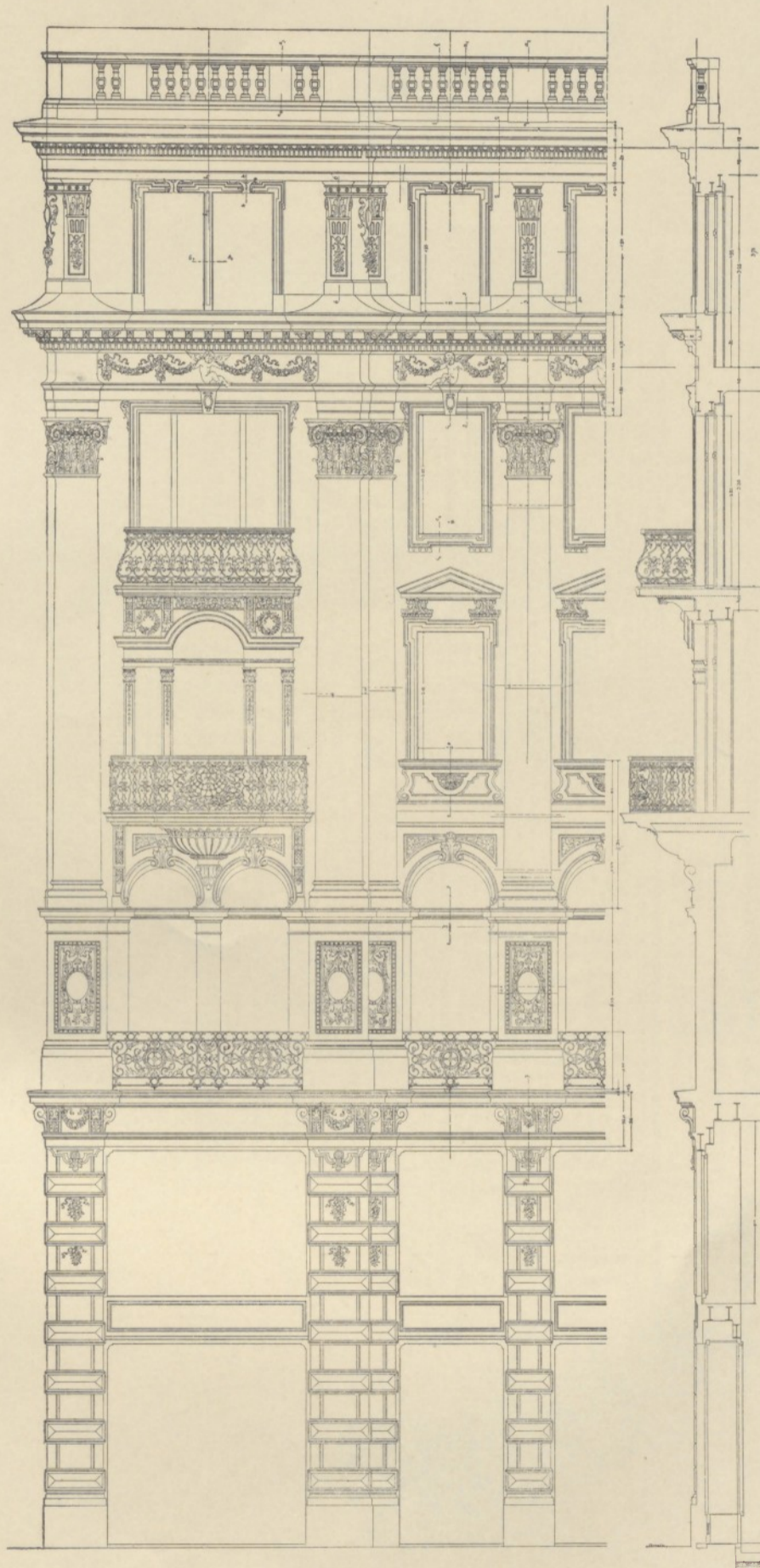
GESCHÄFTS- UND WOHNHAUS IN WIEN, I., TUCHLAUBEN. ARCHITEKT LUDW. RICHTER, WIEN.
