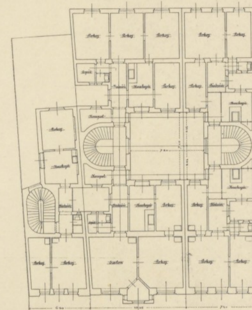
GRUNDRISS DES I. STOCKES.
