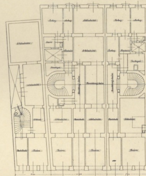
PARTERRE-GRUNDRISS
