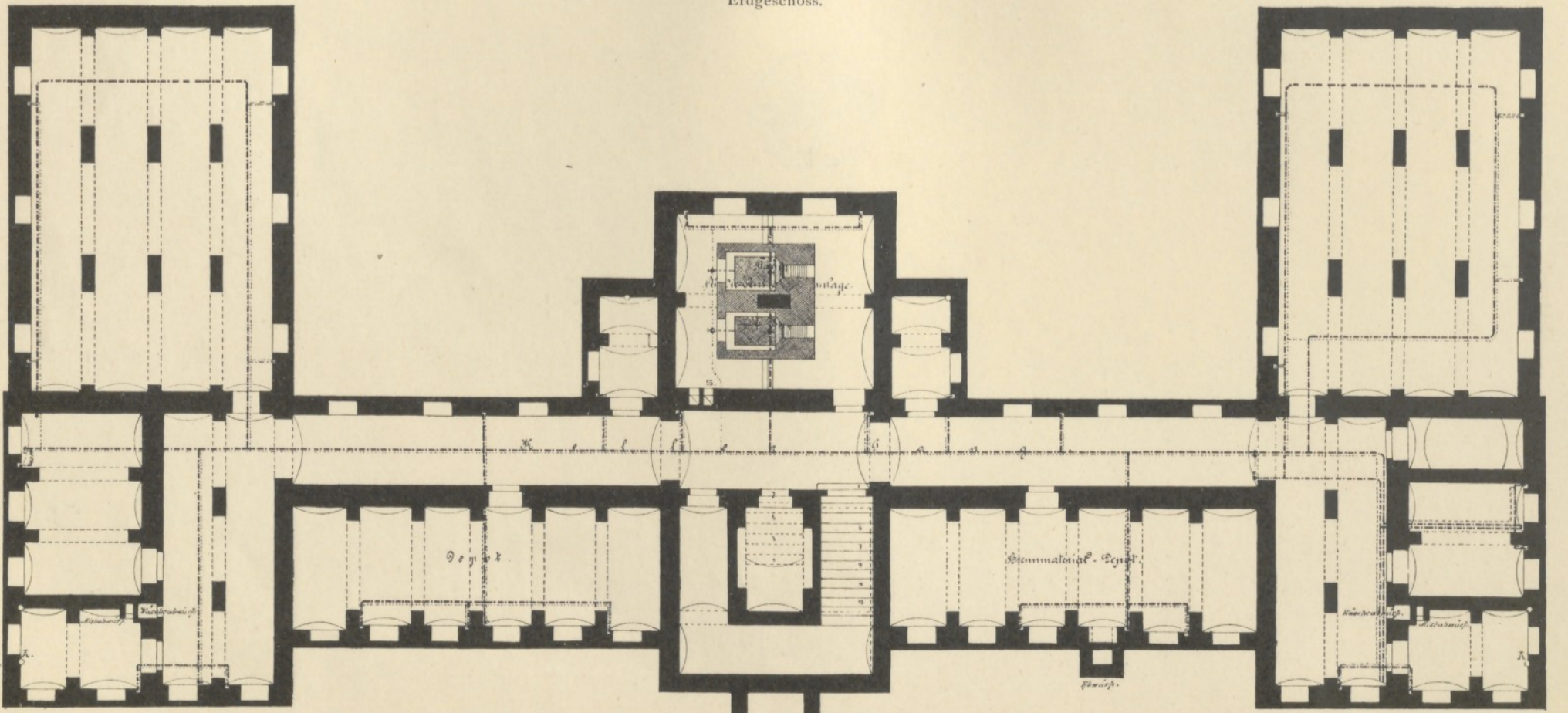
Kellergeschoss.
