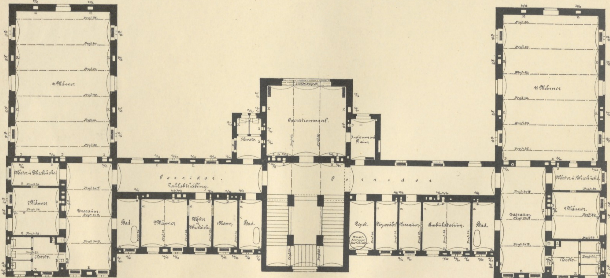
Obergeschoss.
