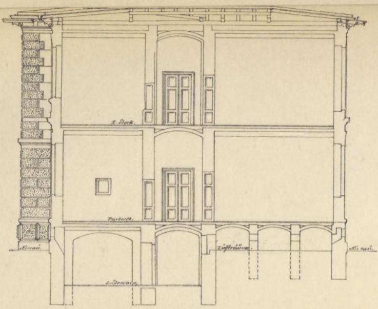
Schnitt.
