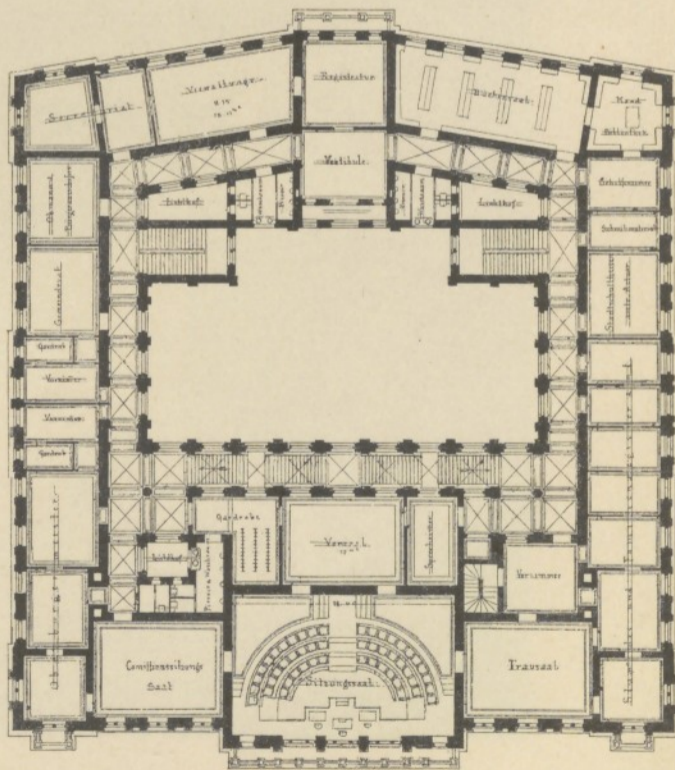
2. Obergeschoss.
