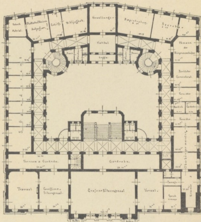
2. Obergeschoss.
