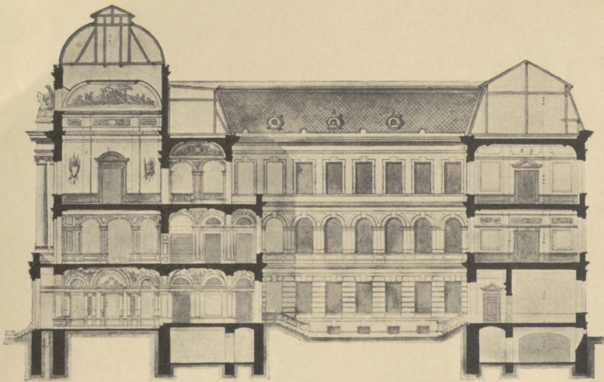
Längsschnitt.
