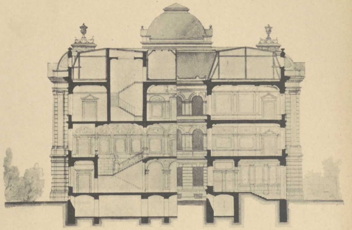
Querschnitt.
