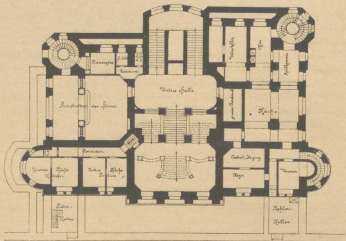
Zweites Souterrain.
