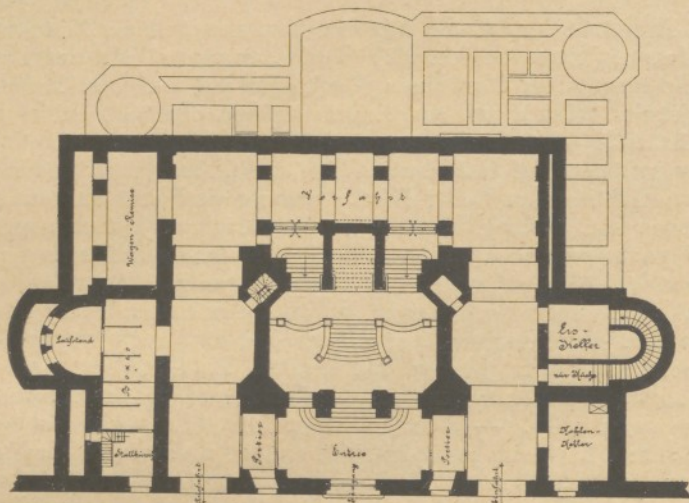
Erstes Souterrain.
