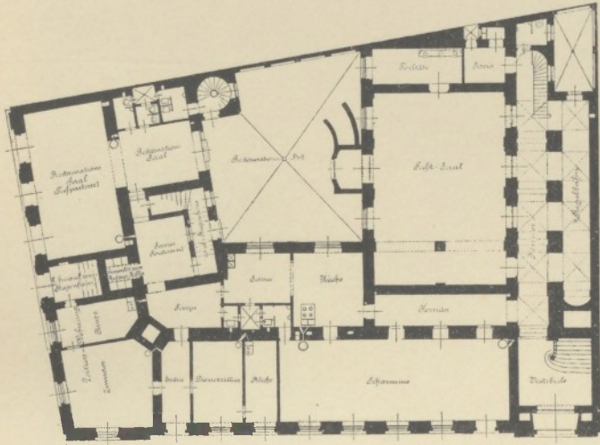
Souterrain und Tiefparterre.
