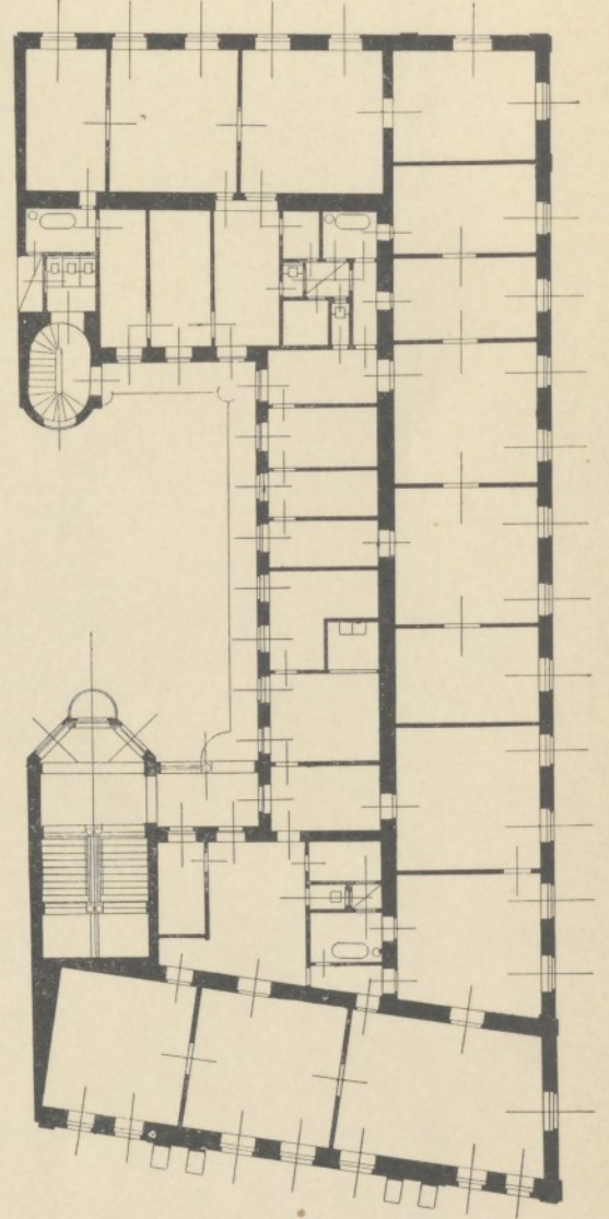
2. Stock: Wohnungen.
