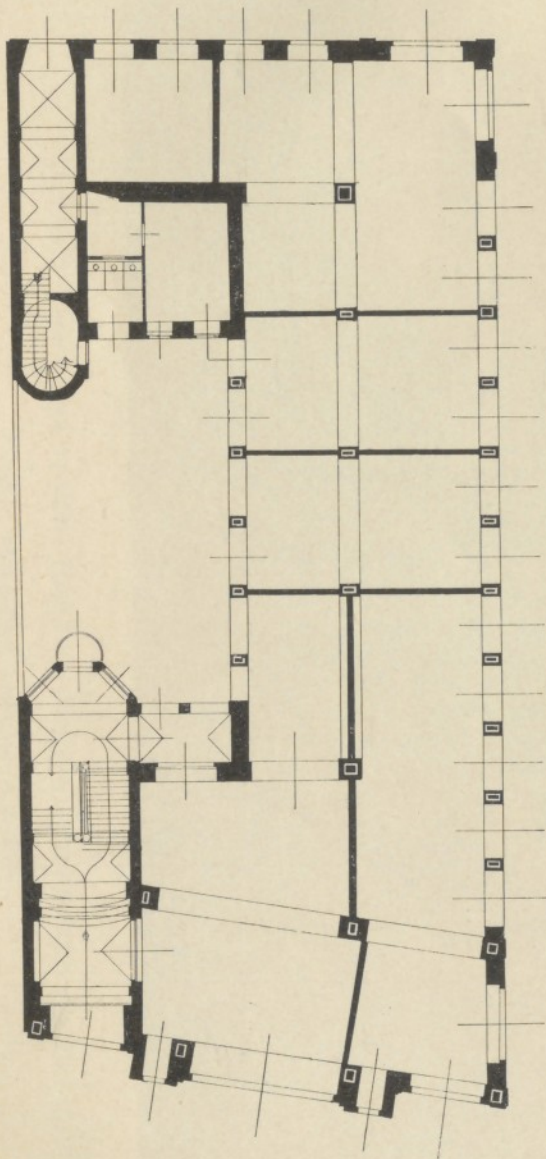
Erdgeschoss: Geschäftslocale.
