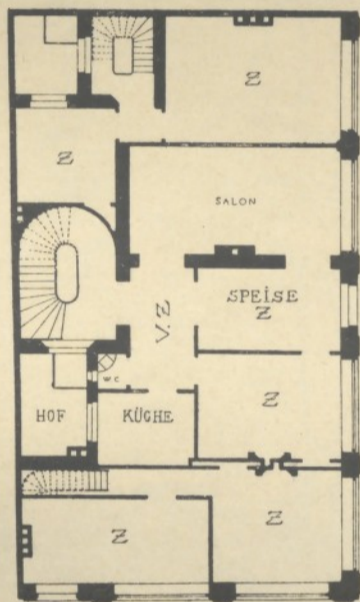
ENTRESOL
