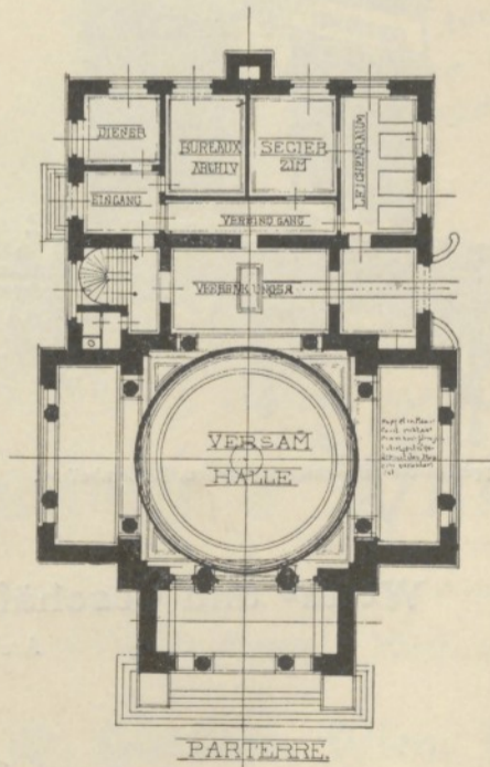
IV. Preis. Grundriss.
