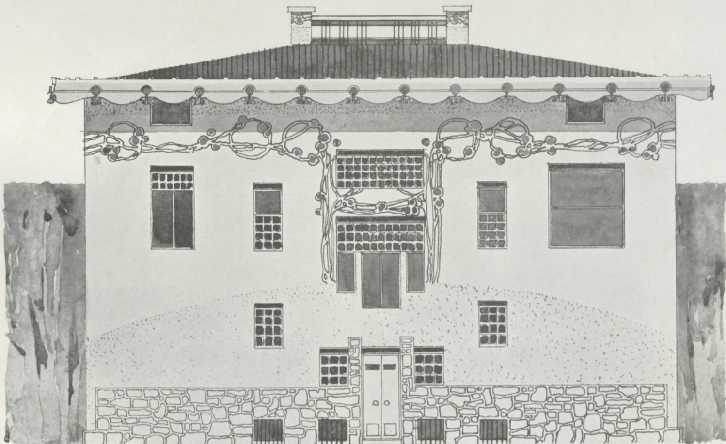
Entwurf für eine Villa. 1. Vorder- und Rückansicht. Seitenansicht und Grundriss im Textblatt.
