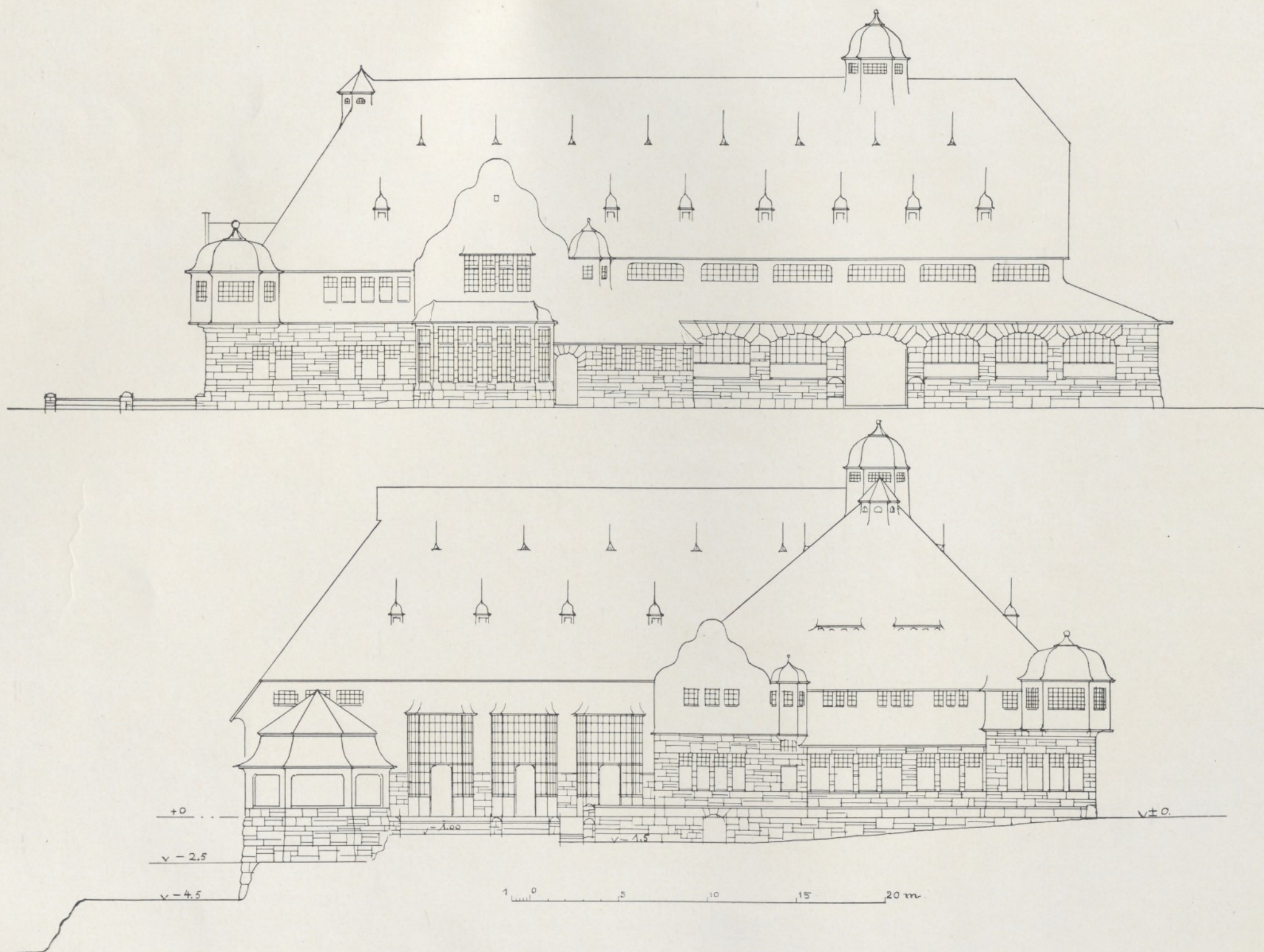
Parkhalle für Remscheid. Grundriss im Textblatt.
