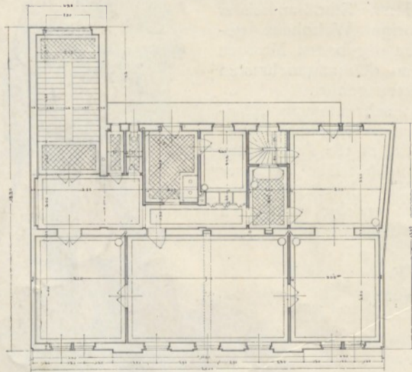
(Grundriss des I. Stockes, zu Tafel 13.)
