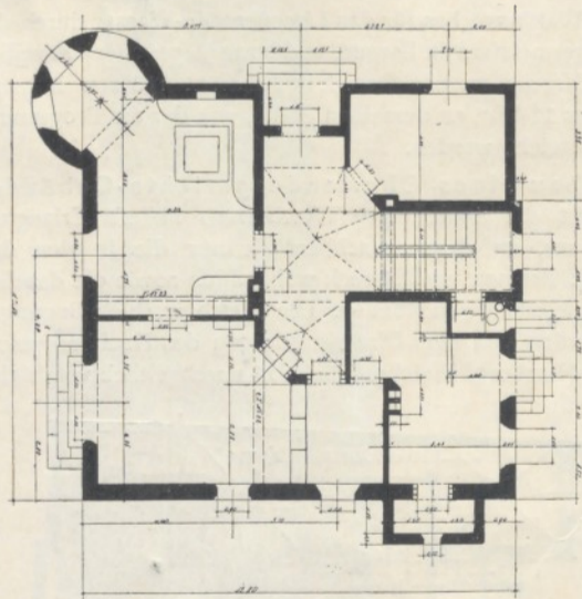
Grundriss zu Tafel 35.
