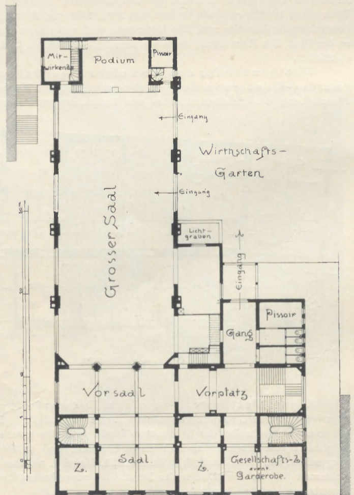
Grundriss zu Tafel 39, 40.
