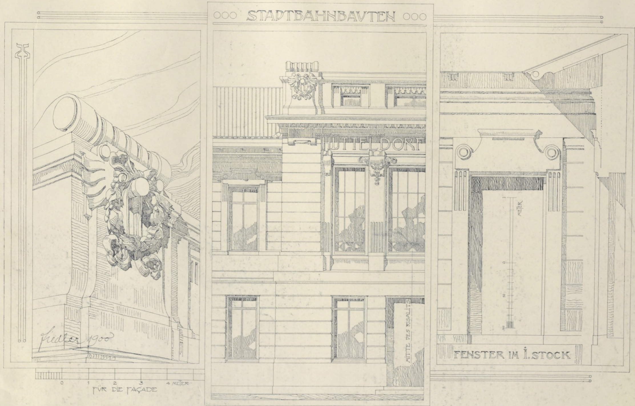
Architekt k. k. Oberbaurath Otto Wagner. STADTBAHNSTATION HÜTTELDORF-HACKING (aus dem neuen Werke: »L. Fiedler, Das Detail in der modernen Architektur«).
