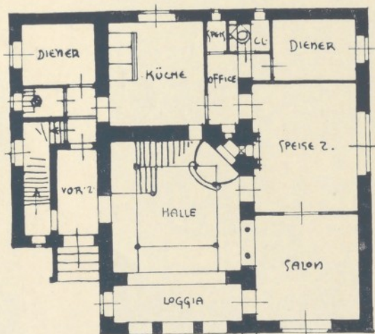
Grundriss des Hochparterre.
