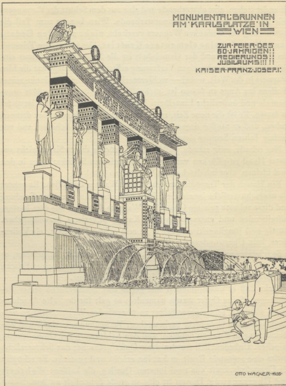
ENTWURF FÜR EINEN MONUMENTALBRUNNEN AM KARLSPLATZ IN WIEN, 1905
