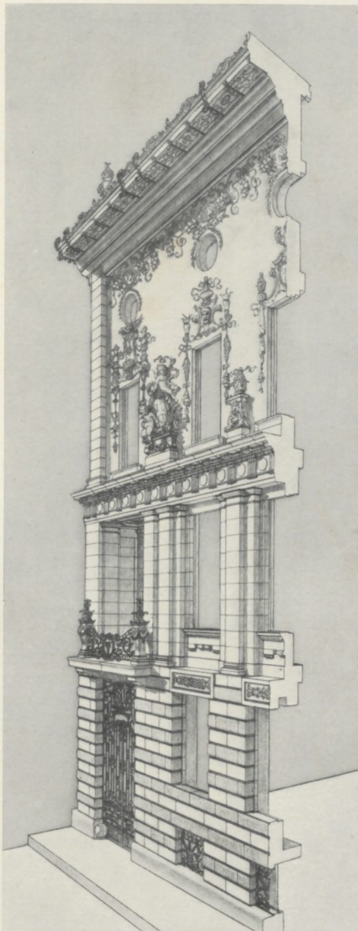
PALAIS OTTO WAGNERS AM RENNWEG WIEN. 1889. FASSADEN-DETAIL
