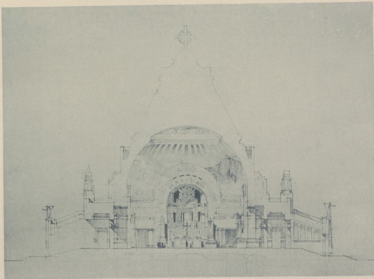
FRANZ MATAUSCHEK. SKIZZE. SCHNITT UND STUDIE ÜBER DEN LICHT-EINFALL DURCH DIE GLASDECKE DER KUPPEL.
