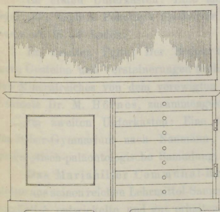
Zerlegbarer Doppel Pultkasten für Mineralien. C Vorderansicht D Seitenansicht.
