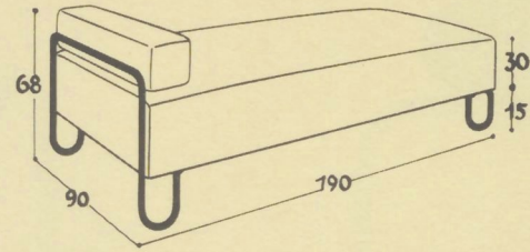
LS 24 THONET Entwurf A. Lorenz
