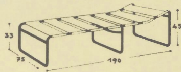
B 15 THONET Entwurf M. Breuer
