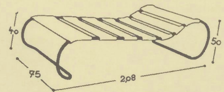
LS 22 Liegestuhl ohne Auflage LS 23 Liegestuhl mit Polsterauflage THONET Entwurf A. Lorenz D. R. G. M. 1154 964
