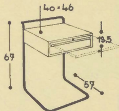
B 117 THONET Internat. Musterschutz Nr. 2569
