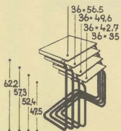
BT 97/100 THONET Entwurf K. Lengyel Musterregister Nr. 39184
