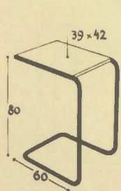
B 118 Var. THONET
