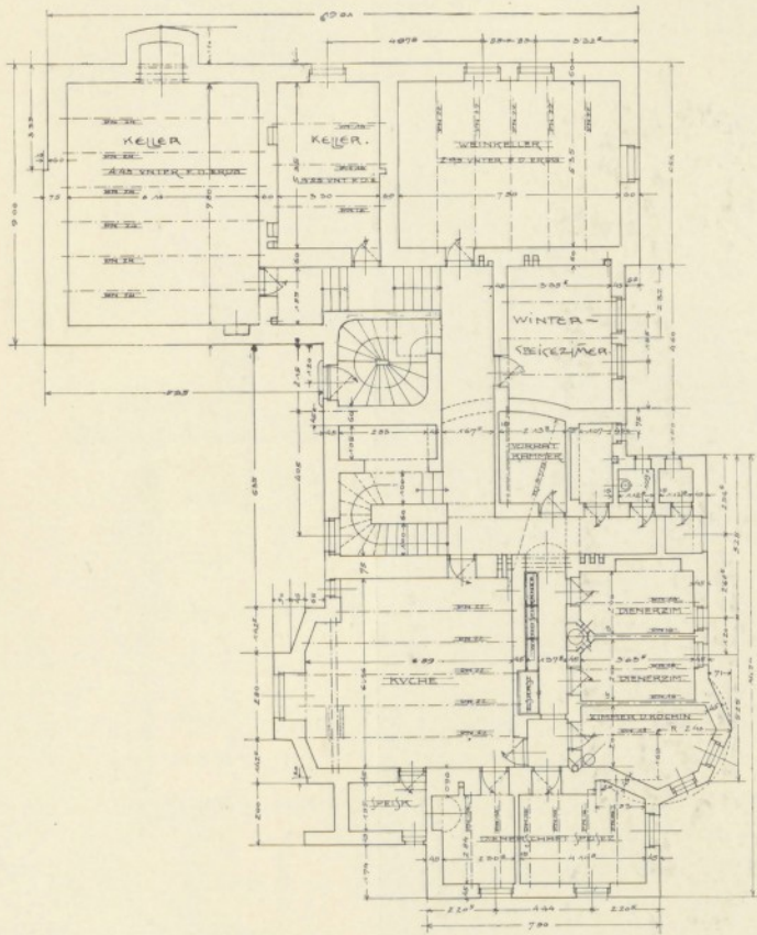
Untergeschoß.
