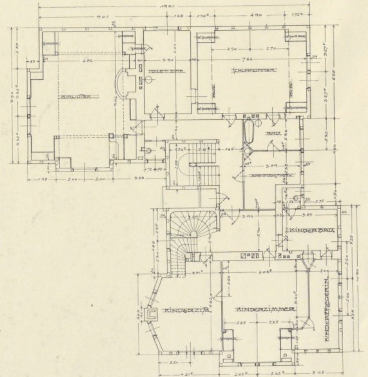
Obergeschoß.
