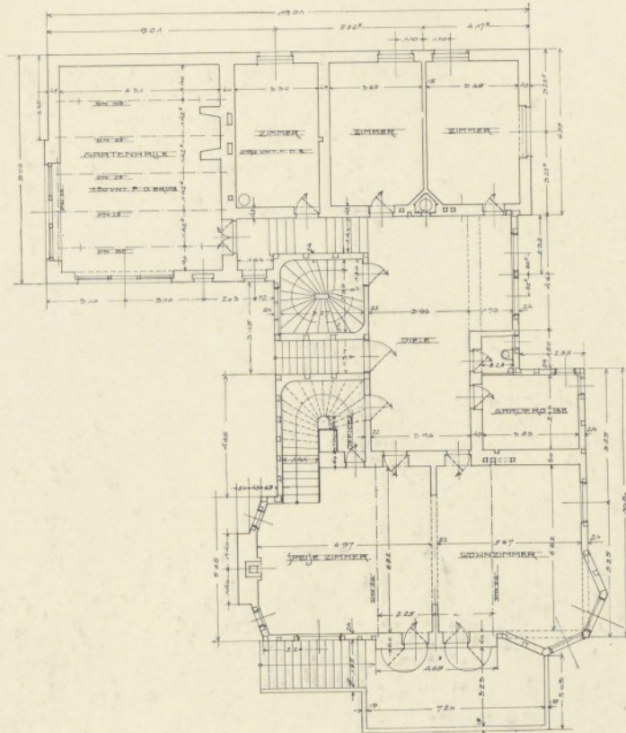
Erdgeschoß.
