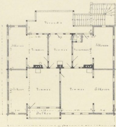
Obergeschoß.
