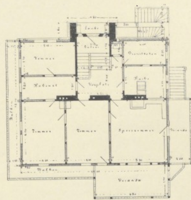
Erdgeschoß.
