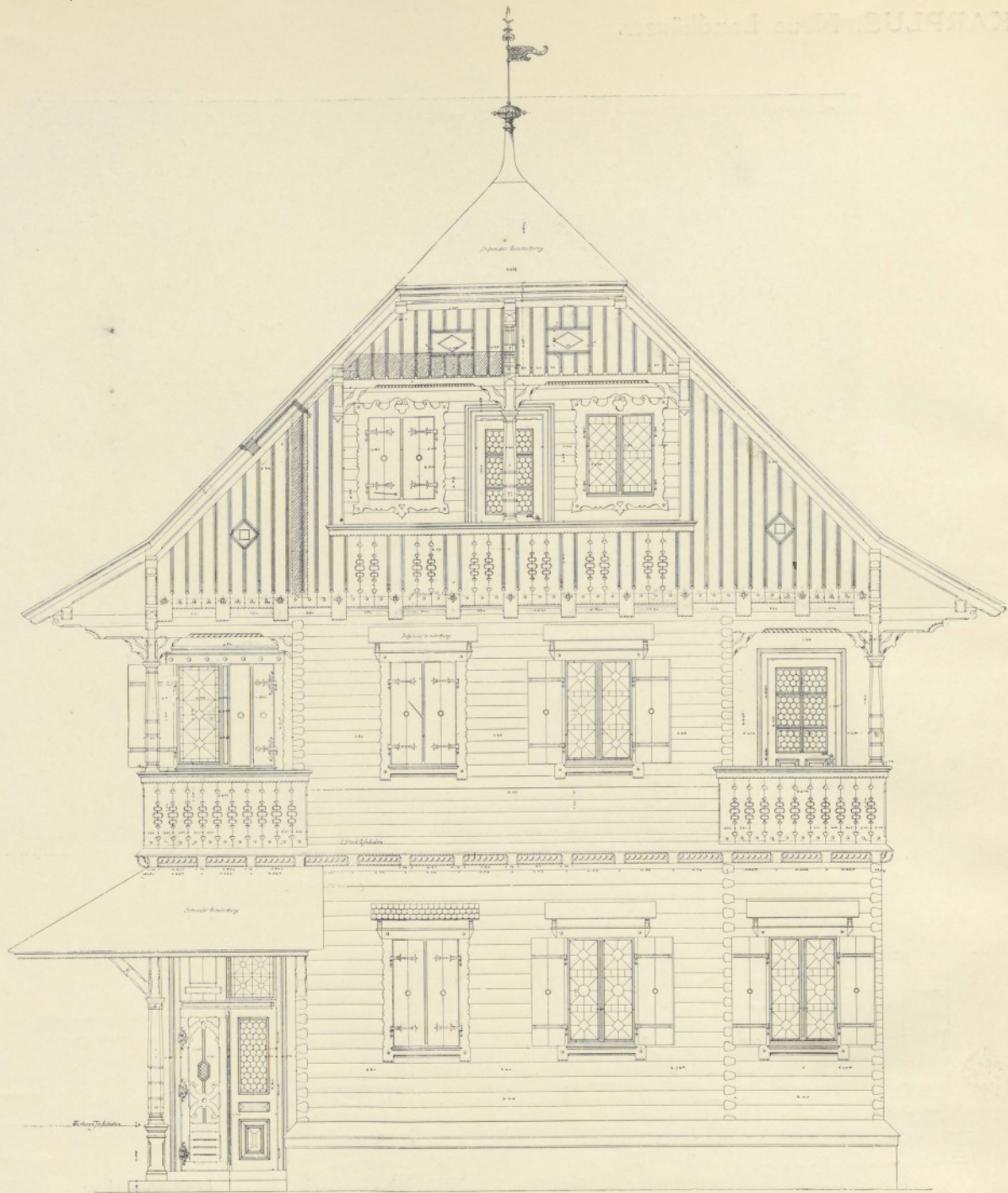
Fassadendetail und Schnitt.
