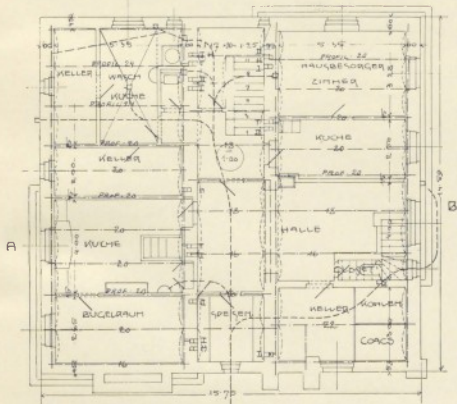
Kellergeschoß.
