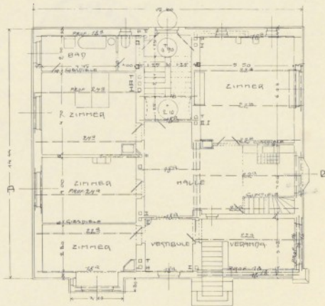
Erdgeschoß.
