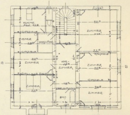
Obergeschoß.
