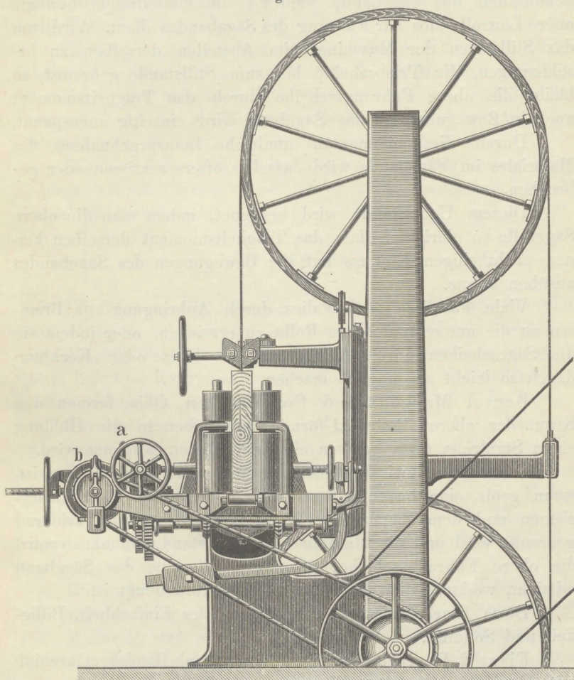
Bandsäge von Richards, London und Kelley. Vorderansicht.
