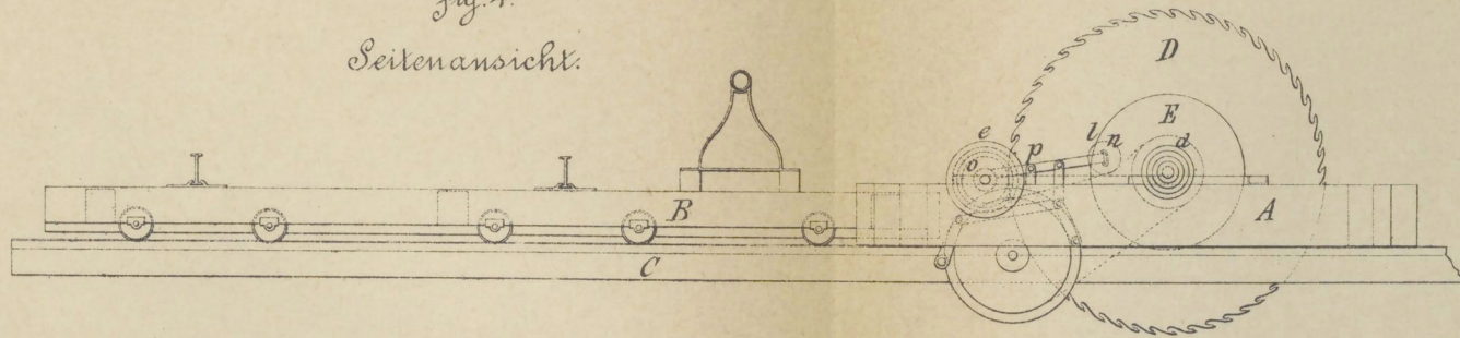
fig. 5. Draufsicht.
