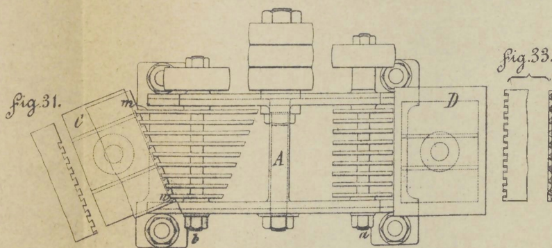
fig. 30. Draufsicht
