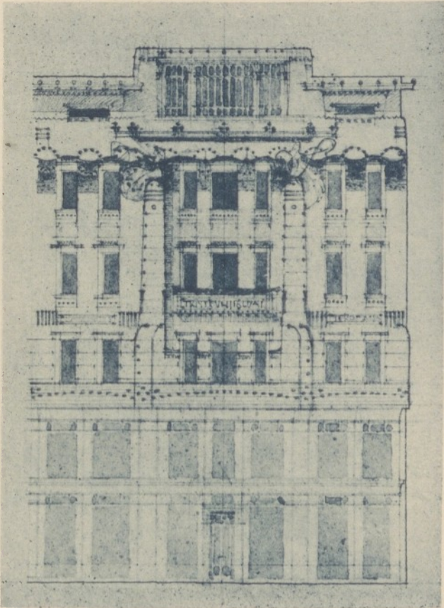
ALBRECHT MICHLER. MIET- UND □ GESCHÄFTSHAUS, FAÇADEN. □ □ SCHULPROJECT. I. JAHRGANG. □
