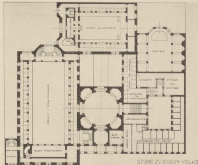
STVDIE ZV EINEM VOLKS- BAD. GRVNDRISS DES I. STOCKWERKS. M. ST. 1:200
