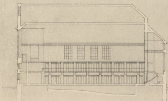
STVDIE ZV EINEM VOLKSBAD. SCHNTT DVRCH DAS MAENNER SCHWIMMBAD. ANSICHT GEGEN DIE SEITE DER VORREINICVNG. IM MASZTAB 1:100. SCHNITT DVRCH DIE VORHALLE 1:200 SCHNITT DVRCH DIE MAENNER SCHWIMMHALLE GEGEN DIE SCHWIMMSEITE. VND DVRCH DEN WANNENBADTRAKT. LAENGSCHNITT DVRCH DIE MAENNERSCHWIMMHALLE.
