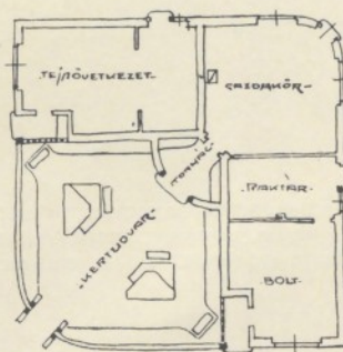
NÉPHÁZAK ÉS GAZDAKÖRI MÉHES. DARÁNYI MEGBÍZÁSÁBÓL MEGALKOTOTT TÍPUSOK. BAUERNCONSUMHÄUSER UND GEMEINDEBIENENZUCHTHAUS, DER „VOLKSHAUS“-TYPUS WURDE VON MIR IM AUFTRAGE DES ACKERBAUMINISTERS DARÁNYI IM JAHRE 1907 KREIERT.
