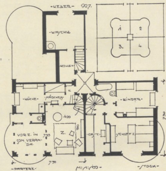
ELSŐ ÉPÍTÉSZETI TERVEM. NÉGYES IKERHÁZ, A 10.000 PENGŐ. MEIN ERSTER ARCHITECTURENTWURF. VIER-ZWILLUNGHAUS, A 10.000 UNG. GULDEN.
