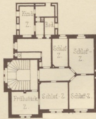
Obergeschoss.
