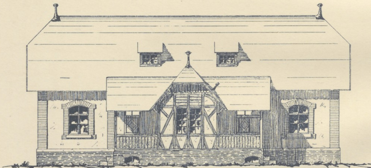
Vorderansicht
