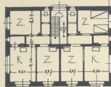
Erdgeschoss
