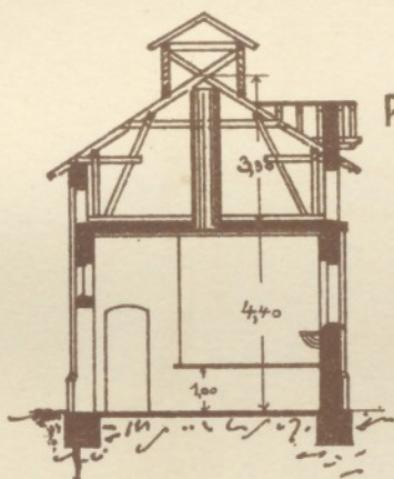
Schnitt A-B.
