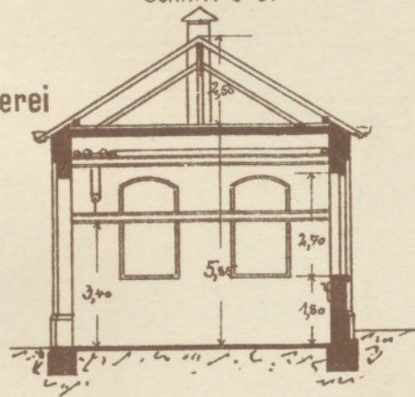
Schnitt C-D.
