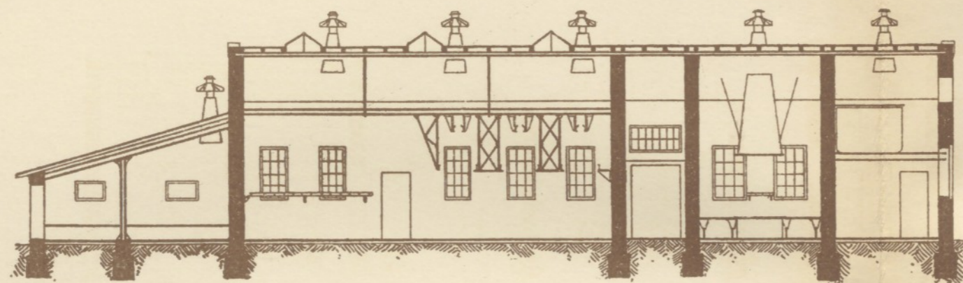
Fig. 6. Längenschnitt durch das Hauptgebäude.
