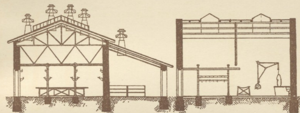
Fig. 7 u. 8. Quer- und Längenschnitt durch die Schweineschlächterei.
