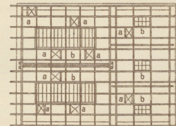
Fig. 10. Sparrenlage.
