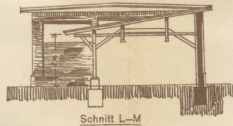
Schnitt L-M
