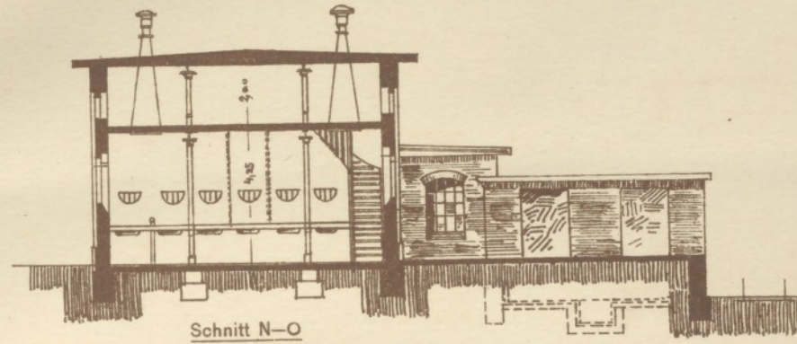
Schnitt N-O
