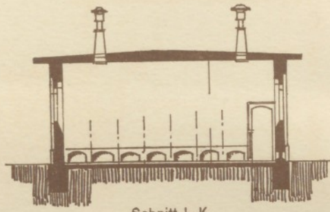
Schnitt I-K
