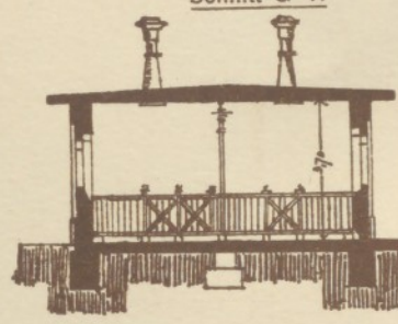
Schnitt G-H
