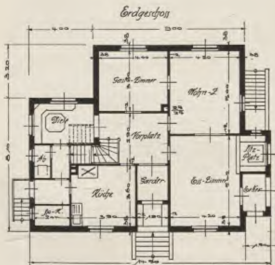
ARCH. BEUTINGER & STEINER, STUTTGART-HEILBRONN ▣ GRUNDRISS ZUM HAUS STRÖBLE IN HEILBRONN
