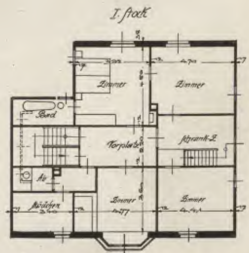
ARCH. BEUTINGER & STEINER, STUTTGART-HEILBRONN ▣ GRUNDRISS ZUM HAUS STRÖBLE IN HEILBRONN
