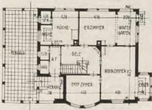
GRUNDRISS ZUM HAUS KOLB (VGL. S. 44)
