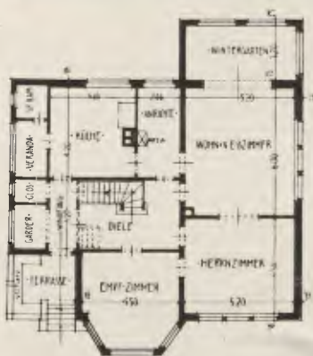
HAUS DR. ALBERT BEITTER IN GÖPPINGEN STRASZENSEITE U. GRUNDRISS VON ERD- UND OBERGESCHOSZ (BAUKOSTEN: 36 000 M.)
